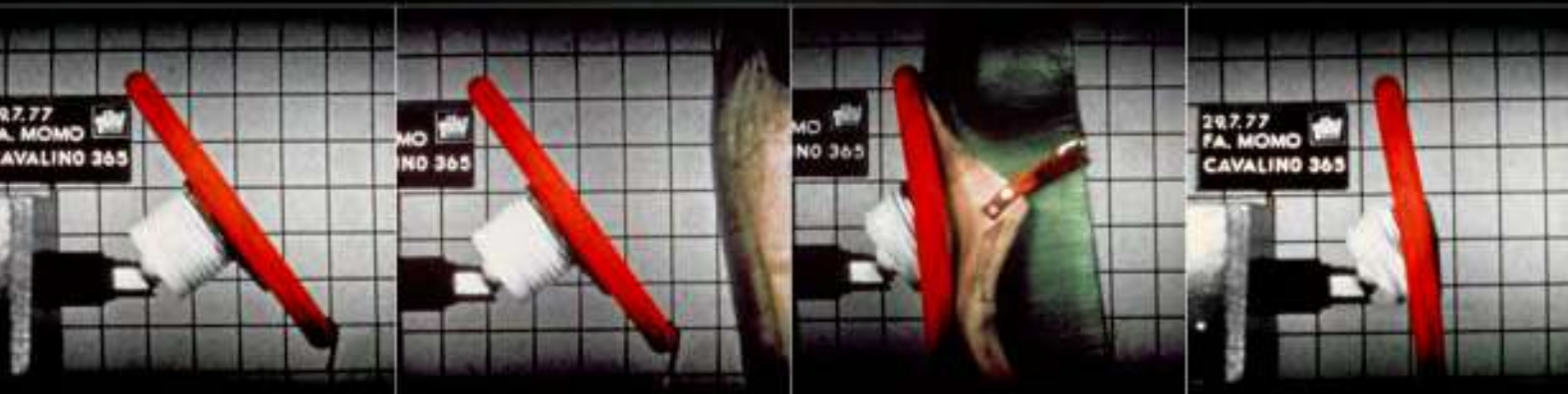
Impact test of the "dummy" against the assembly: wheel-hub-car, shows a perfect interaction of energy absorbtion forces. Prove d'urto del manichino contro il sistema "volante-mozzo-vettura", dimostrano un'efficiente interazione degli assorbimenti di energia.
